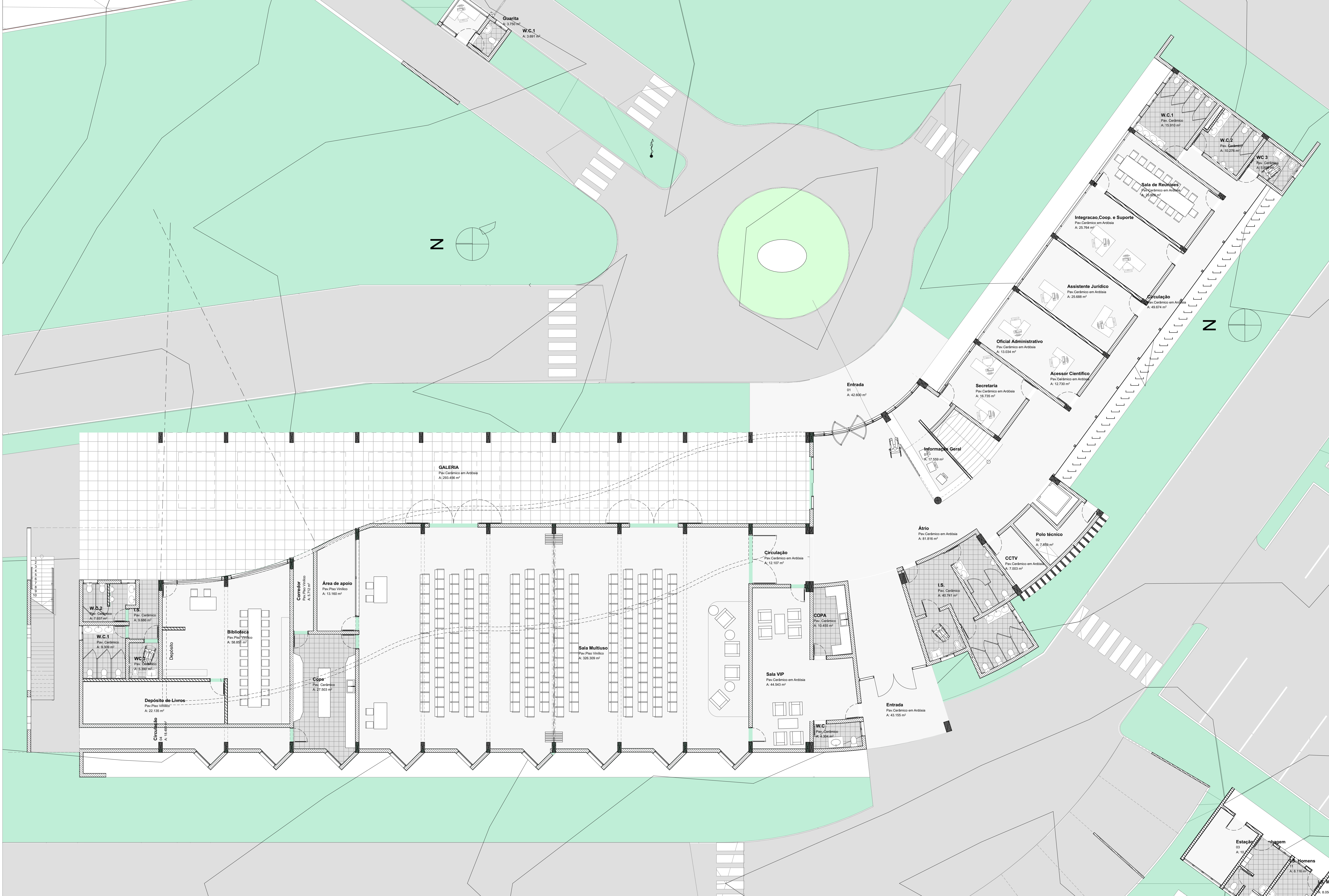
0. PISO 1 - COMPLETO 1:100
