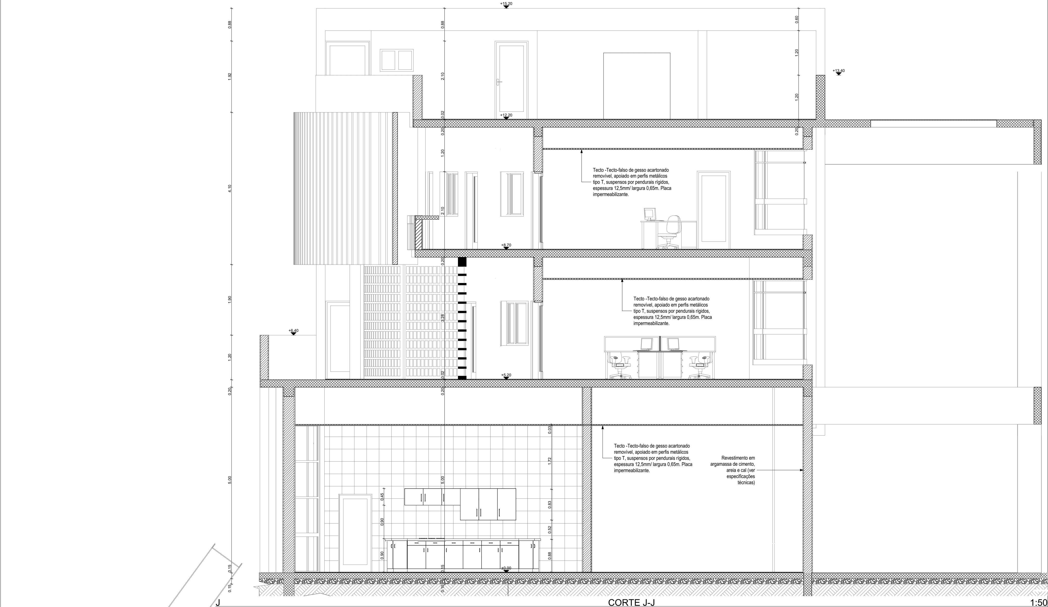
CORTE J-J
